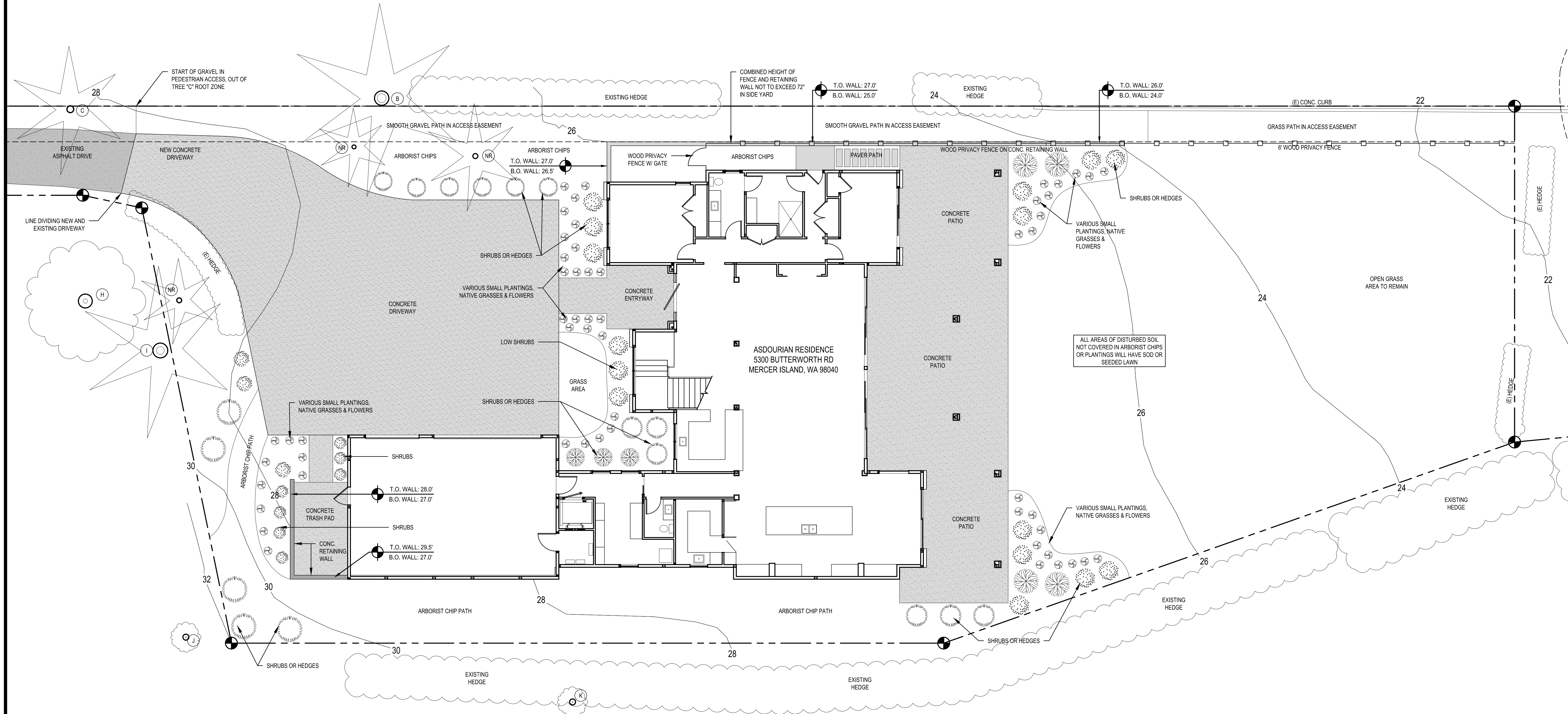
1 LANDSCAPE PLAN SCALE: 1/8" = 1'-0"
